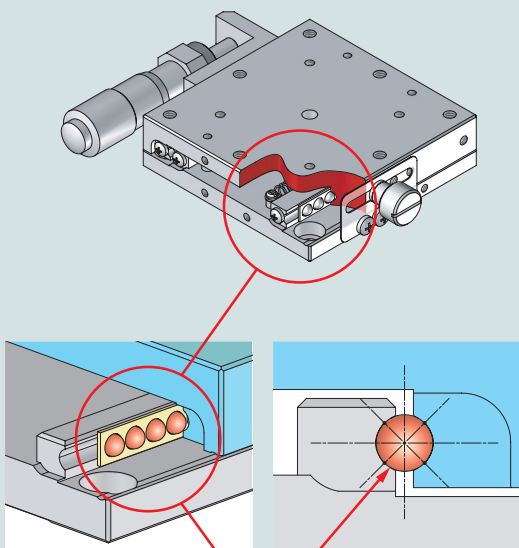
哥特式圓弧槽 (4點結構)
